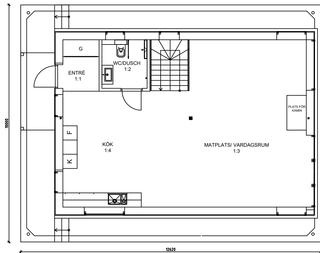
PLAN 1 ENTRÉPLAN, ca 74kvm+ Däcksyta ca 37.3 m 2 SKALA 1:100
