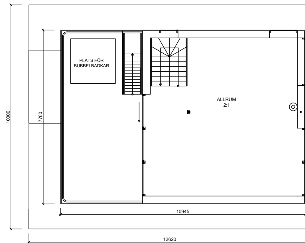
PLAN 2 ÖVERPLAN, ca 48kvm + Takyta/terrass ca 22kvm SKALA 1:100
