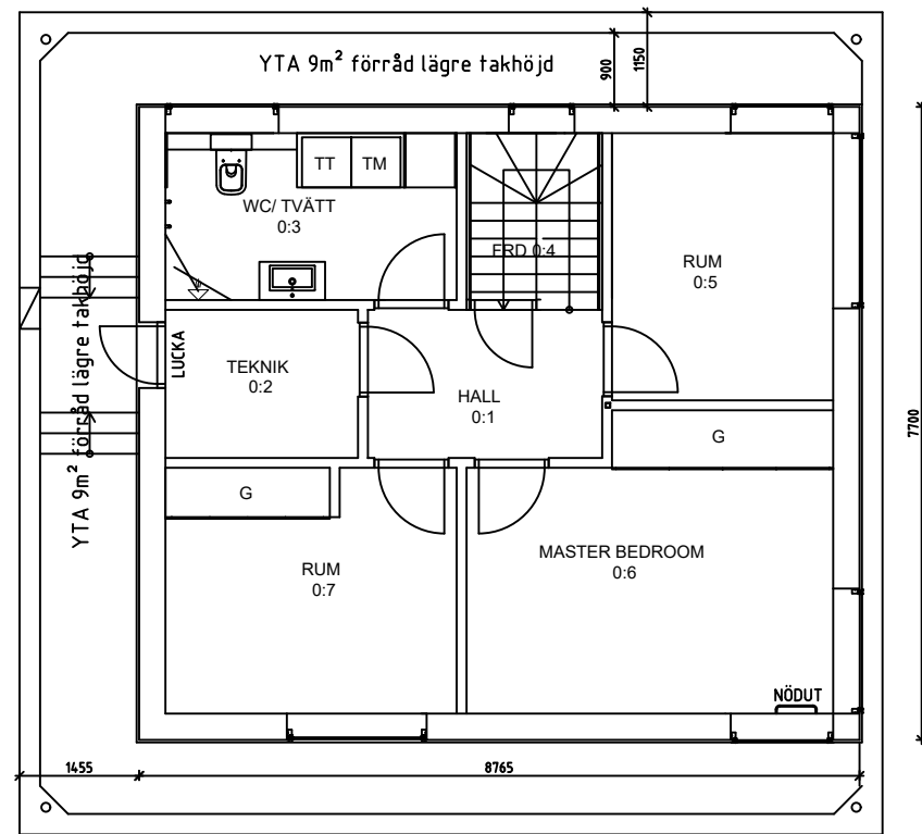
PLAN 0 KASSUNPLAN, 58 kvm + KALLFÖRRÅDSYTA 26 kvm SKALA 1:100
