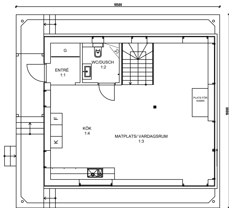
PLAN 1 ENTRÉPLAN, 58kvm+ Däcksyta 32 m 2 SKALA 1:100
