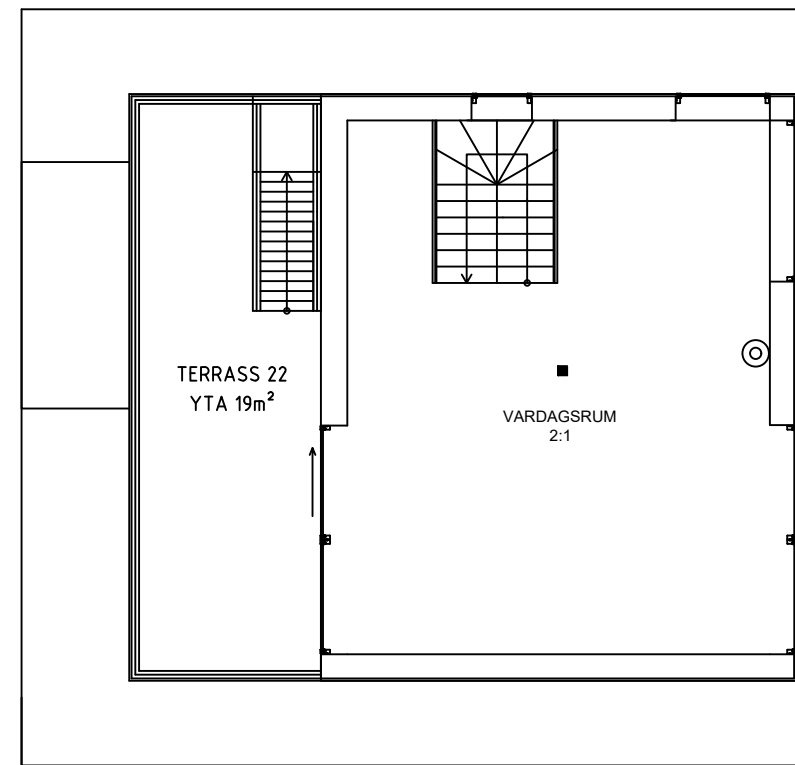
PLAN 2 ÖVERPLAN, ca 41kvm + Takyta/terrass ca 19kvm SKALA 1:100
